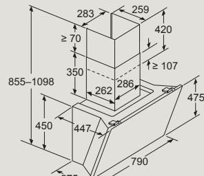
Gerät im Abluftbetrieb
