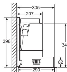
Montage bei Geräten mit Absenkrahmen - Möbelkorpus-tiefe laut Kombinationstabelle
