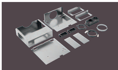
LZ21WWM11 Einbausatz Montageset für abnehmbare Lüfter
