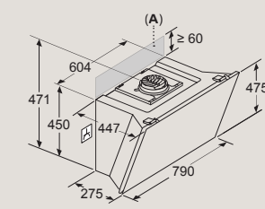
Gerät im Umluftbetrieb ohne Abluftkanal
