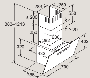
Gerät im Umluftbetrieb
