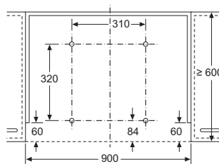
Montage Flachschirmhaube mit Absenkrahmen Montage direkt an der Küchenwand
