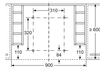
Montage Flachschirmhaube mit Absenkrahmen Möbel mit seitlichen Regalfächern Montage direkt an der Küchenwand
