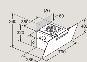
Gerät im Umluftbetrieb ohne Abluftkanal
