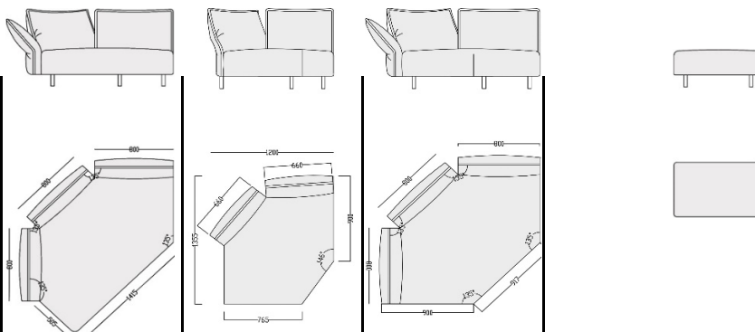
Trapezelement trio zum einseitigen Anbauen
